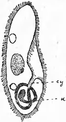
Рис. 2. Инфузория Туфелька в растворе хлористого магния: су—глотка, к—тушевая „кишка“ (по Догелю).
