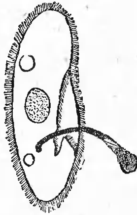
Рис. 3. Инфузория Туфелька, при помещении в слабый раствор серпикислого железа претерпевает процесс обратного выведения пищи—процесс, аналогичный рвоте (по Догелю).
